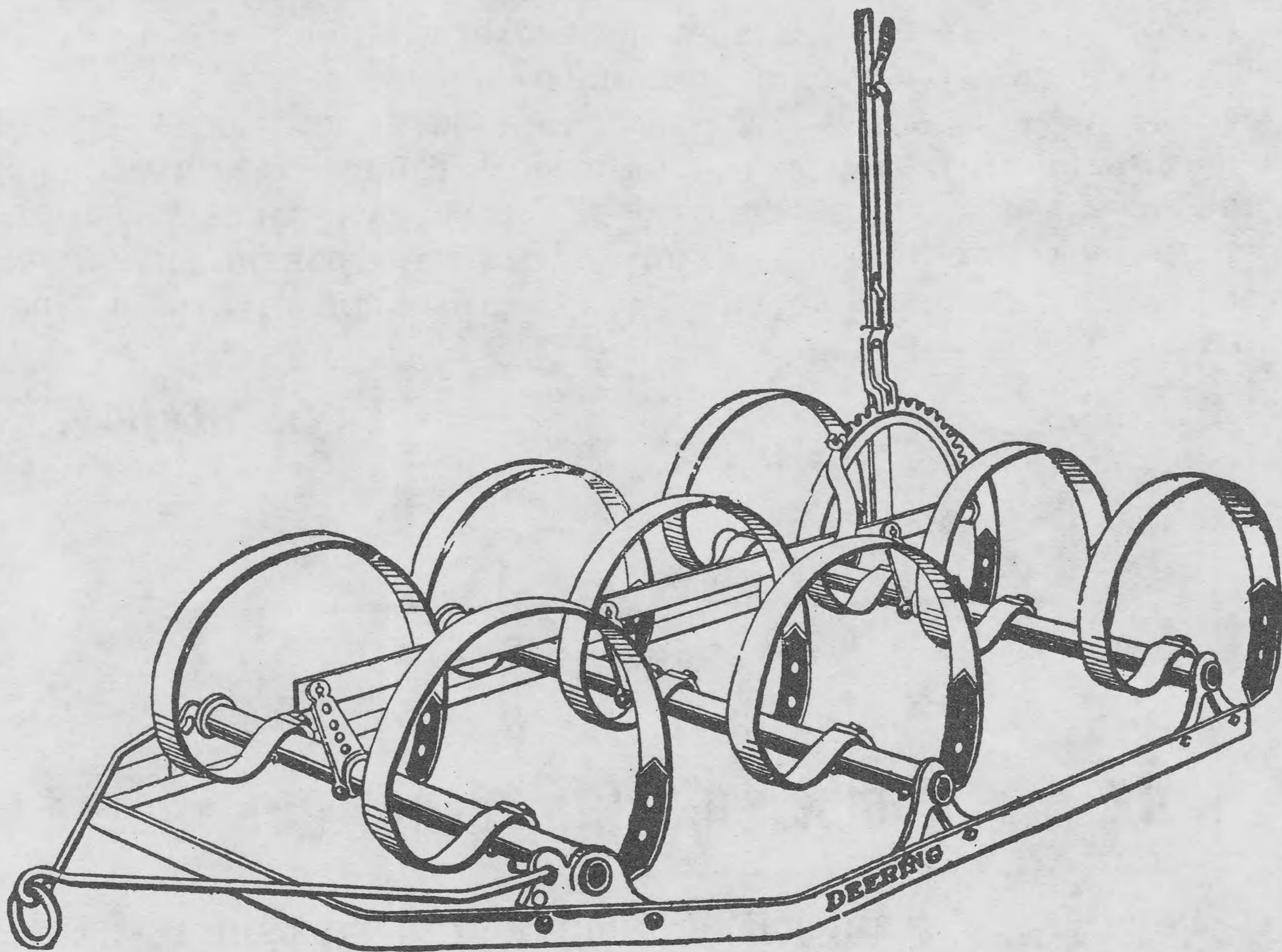
Амэрыканская спрунжыновая барана з 9 зубамі. Такую барану пускаюць па асушэным тарфяным балоце, каб разрыхліць верхні слой.
