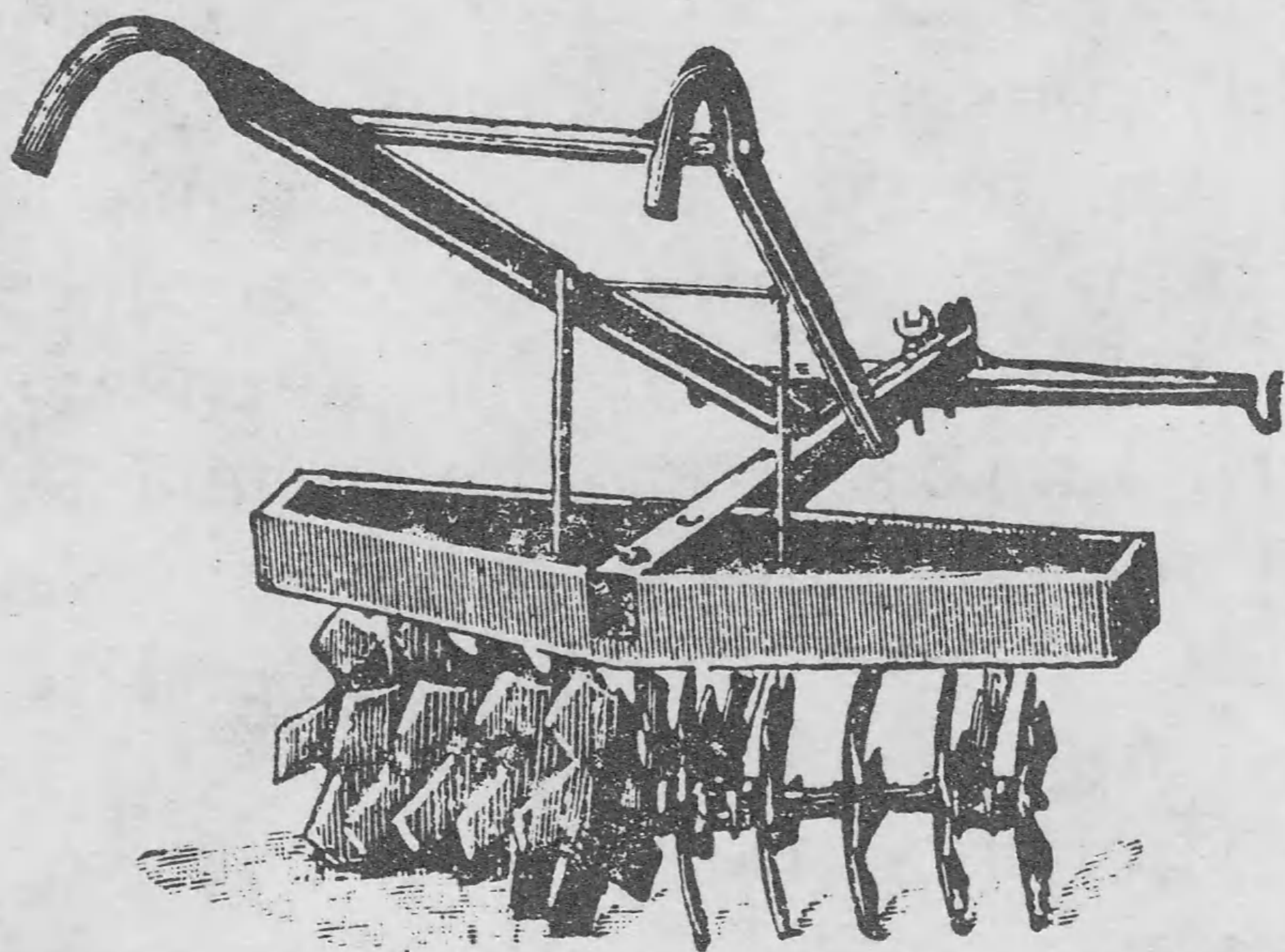
Кальцавая барана з 8 кругамі. Такую барану пускаюць каб парэзаць дзірван.
