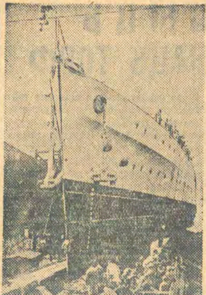
Новы англіскі крэсер. 20 жніўня ў Портсмуте быў спуска на воду новы англіскі крэсер «Аврора», валазшчым у 3.000 тон. Крэсер будзе ўзброены пачынаючы 15-сантыметровымі гарматамі. НА ЗВЯЗДА: спуск на стапелу крэсера «Аврора».
