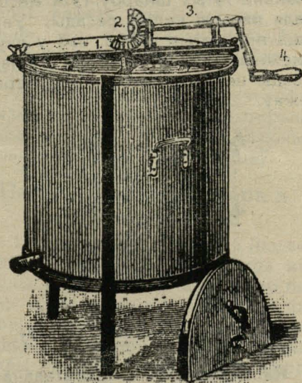
Рыс. 2. Простая мёдагонка з шрубавой корбай. 1 — верхняя прыкрыўка; 2 — конусавідны шруб да корбы, 3 і 4 — корба.
