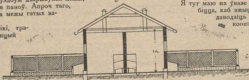
Праэкт трусятніка ў разрэзе
