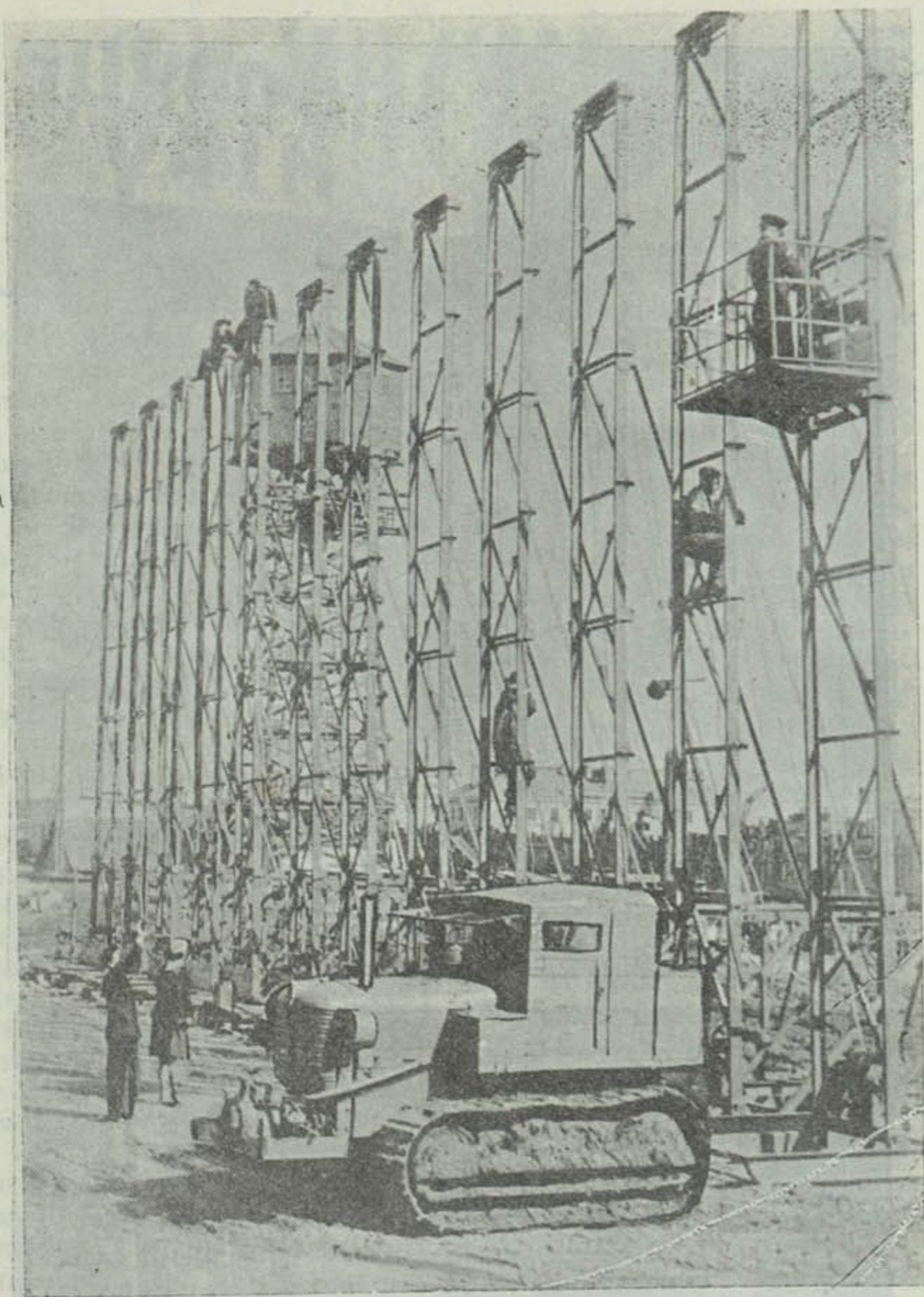
Монтаж мачтавых пад'ёмнікаў для «Куйбышэўгідрабуда» на Нова-сібірскім заводзе будаўнічых машын. (Фотахроніка ТАСС)
