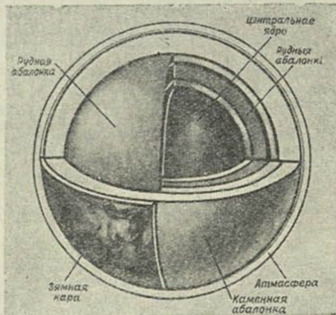
Будова зямнога шара ў разрэзе. У сярэдзіне — цэнтральнае ядро радыусам у 3470 кілометраў. Над ім ляжыць рудная абалонка, яе пакрываюць слаі каменнай абалонкі. Апошні слой прадстаўляе сабой зямную кару. З паверхні зямны шар пакрыты паветранай абалонкай — атмасферай.
