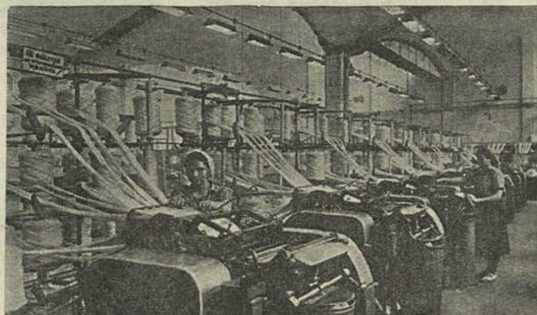
На Мінскім камвольным камбінаце ўступілі ў строй цэхі першай чаргі: часальны, прадзільны, грэбенечасальны і роўнічны. Выдана першая прадукцыя пражы. На здымку: лінія станкоў грэбенечасальнага цэха.
