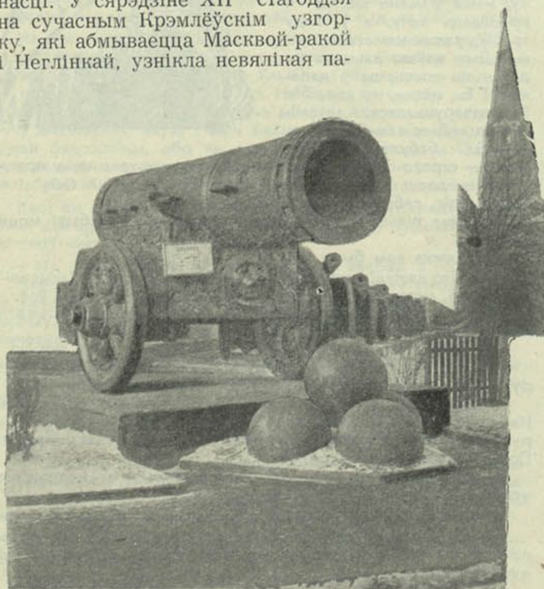
На здымку: цар-гармата. Яна прызначалася для абароны Крэмля і доўгі час знаходзілася на Чырвонай плошчы, недалёка ад Спаскіх, галоўных варот крэпасці. У XIX ст. гармату перанеслі ў Крэмль. Яе лафет і ядры дэкаратыўныя. Вага — 40 тон (бронза), калібр — 890 мм.
