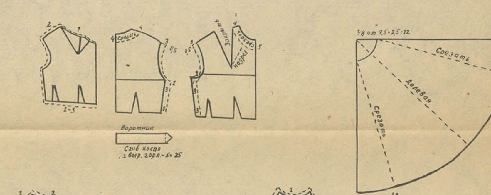
Платье 2. Платье отрезное по линии талии, «японка». На основную выкройку лифа наносят построение «японки» и линии фасона. Юбка из четырех клиньев. Клин выправляют, как показано на рисунке.
