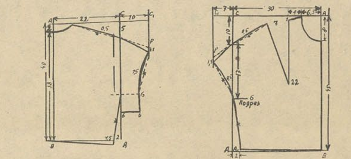
Моделирование Платье 1. Платье цельнокроеное, неотрезное по линии талии. На основную выкройку платья наносят линии этого фасона. По линиям фасона выкройку разрезают и надрезают, внизу по надрезам раздвигают.
