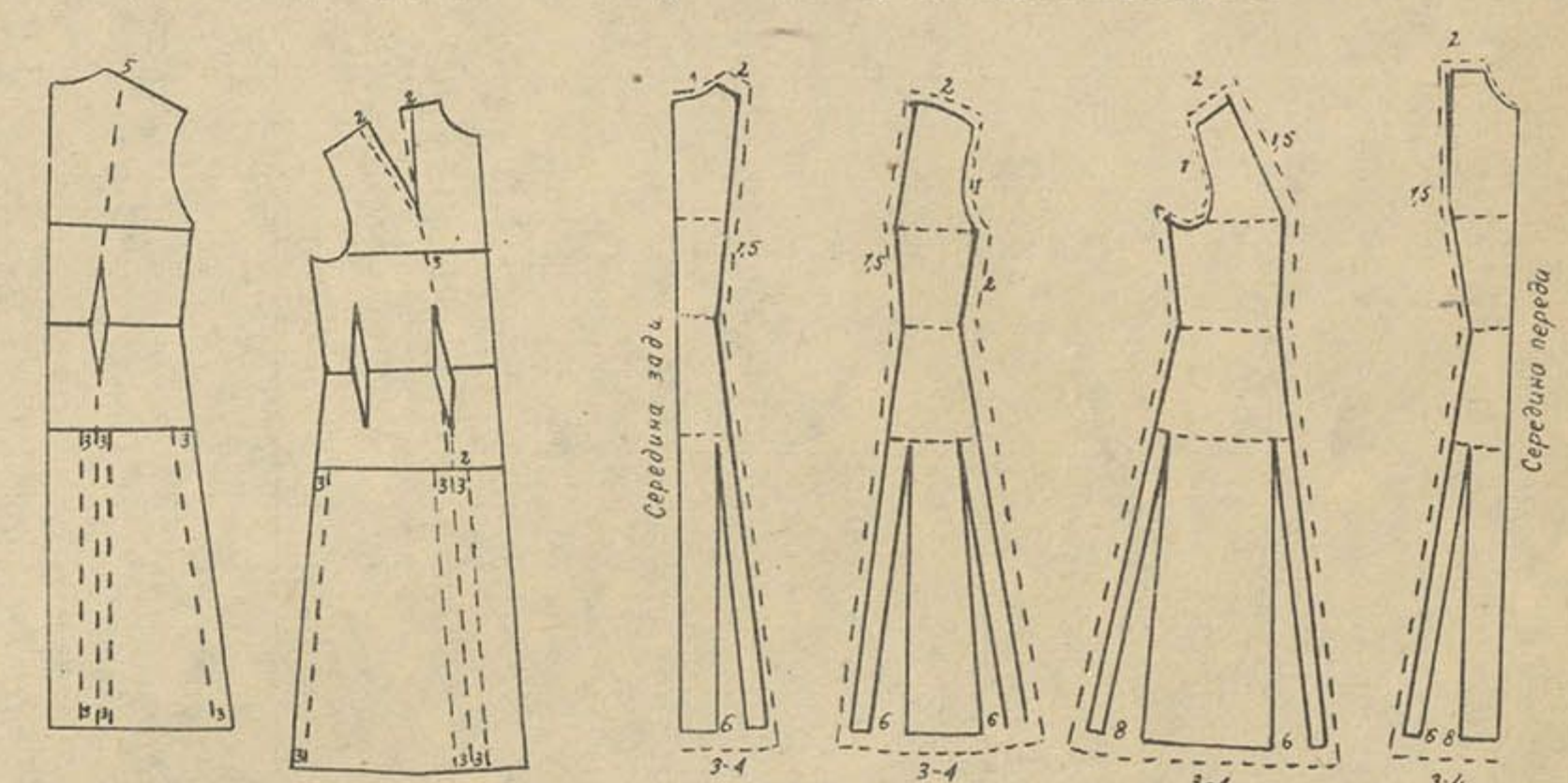
Платье 2. Платье отрезное по линии талии, «японка». На основную выкройку лифа наносят построение «японки» и линии фасона. Юбка из четырех клиньев. Клин выправляют, как показано на рисунке.
