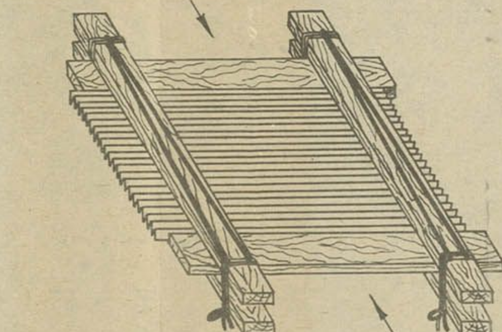
Рис. 6. Форма для гофрирования, зажатая планками. Перед запариванием внутренние планки сдвигают в направлении стрелок.
