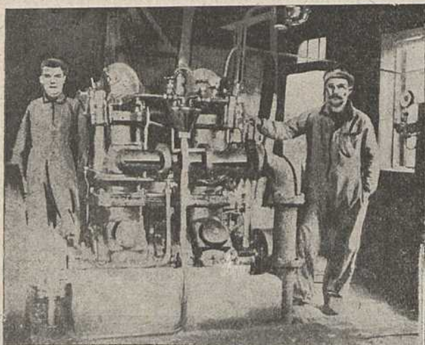
Нафтавы дызэль саўгасу Лапухі-Старыца (36 конскіх сіл) прыводзіць у рух млын, крупазэрку і пільню.
