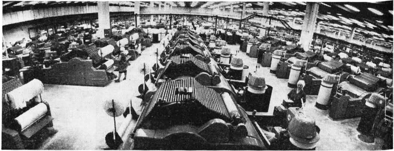
На бавоўнапрадзільнай фабрыцы Гродзенскага прадзільна-нітачнага аб'яднання задзейнічаны 32 новыя кордачасальныя машыны румынскай фірмы «Унірэа». Яны ў 2—2,5 раза больш прадукцыйныя за існуючыя, дазволілі значна палепшыць якасць прачосу і ўмоў працы. Зманціравана і абката на абсталяванне румынскімі і савецкімі спецыялістамі. НА ЗДЫМКУ: участак новых кардачасальных машын.
