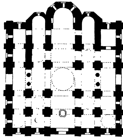
Плян катэдры св. Сафіі ў Полацку паводля І. М. Хозерава.
