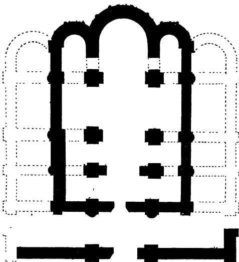
Плян Барыса-Глебскае царквы на Сьмядыне ў Смаленску.
