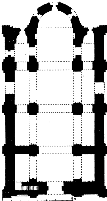
Плян царквы Дабравешчаньня ў Віцебску паводля А. М. Паўлінава.
