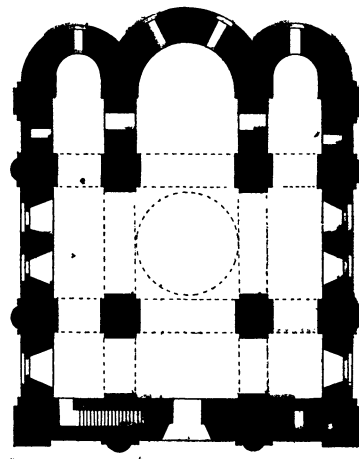
Плян Пятра-Паўлаўскае царквы ў Смаленску паводля І. М. Хозерова.
