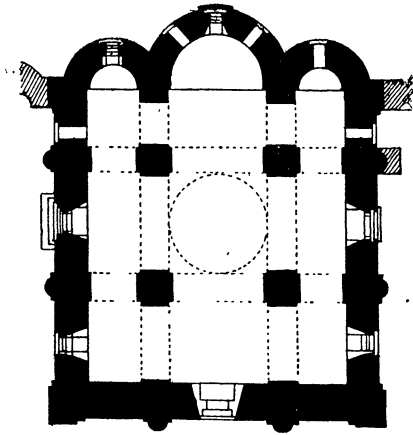
Плян царквы сьв. Івана Багаслова ў Смаленску паводля І. М. Хозерова.
