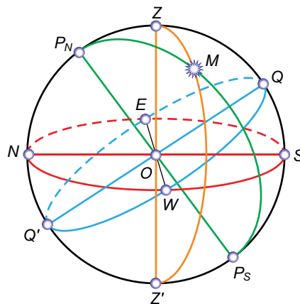
Рыс. 12. Нябесная сфера:
