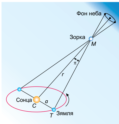
Рис. 122. Паралактычнае зрушэнне зоркі на працягу года: C — Сонца; M — зорка; a — паўвось зямной арбіты; \pi — гадавы паралакс
