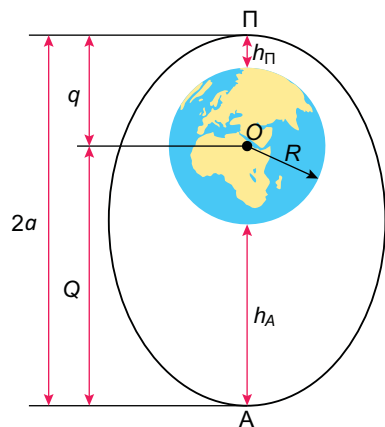
Рыс. 46. Эліптычная арбіта штучнага спадарожніка Зямлі
