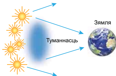
Рыс. 153. Цёмная туманнасць засланне святло зорак, якія знаходзяцца на вялікай адлегласці ад Зямлі
