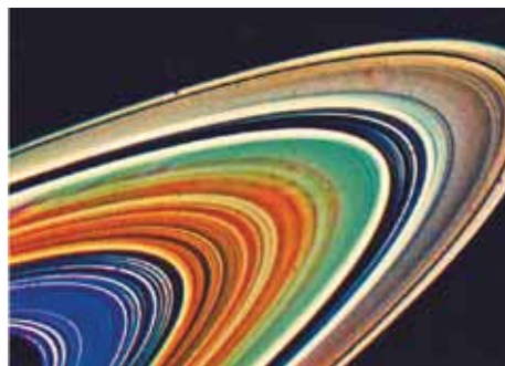
Рыс. 68. Структура кольцаў Сатурна (кольеры ненатуральныя — яны падкрэсліваюць адрозненні мінералагічнага складу кольцаў)
