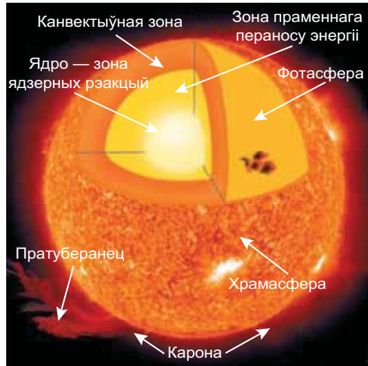
Рис. 110. Будова Сонца
