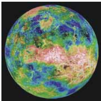
Рис. 57. Рэльефная карта паверхні Венеры, складзеная паводле даных радыёлакацый- ных даследаванняў касмічнага апарата «Магелан»
