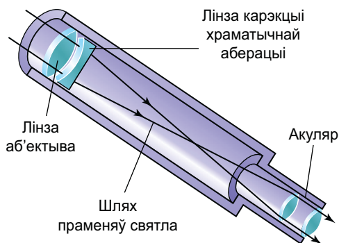
Рыс. 97. Ход прамяняў у тэлескопе-рэфрактары
