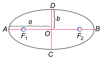
Рис. 37. Элементы эліпса
