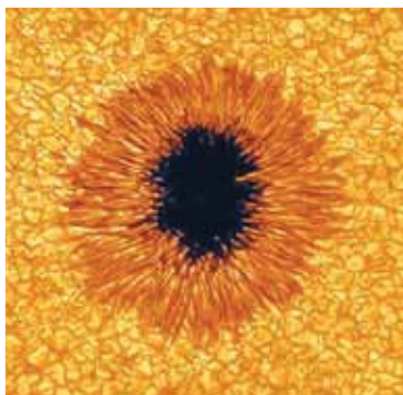
Рыс. 114. Сонечная пляма і фотасферная грануляцыя
