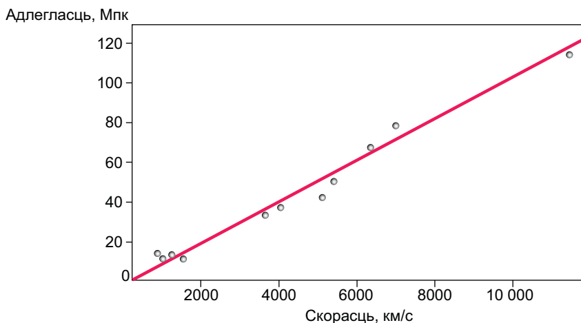
Рис. 161. Залежнасць скорасці аддалення галактык ад адлегласцей да іх
