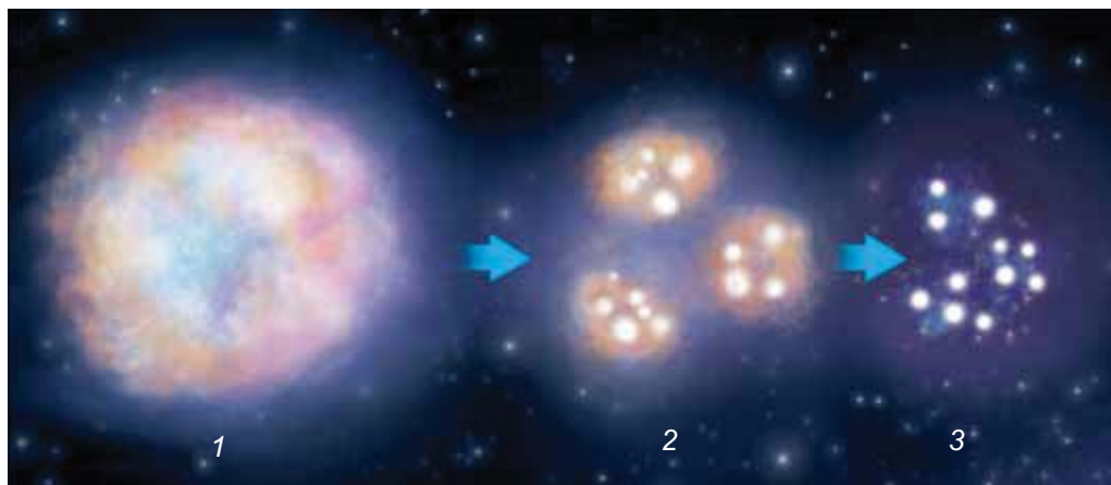
Рыс. 129. Утварэнне зорак з газапылавага комплексу
