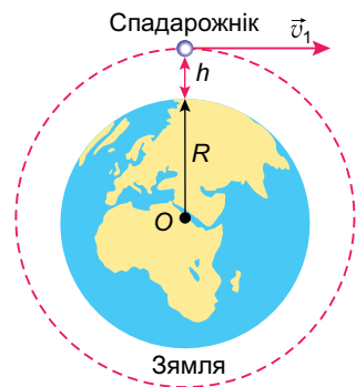
Рис. 45. Рух спадарожніка па кругавой арбіце
