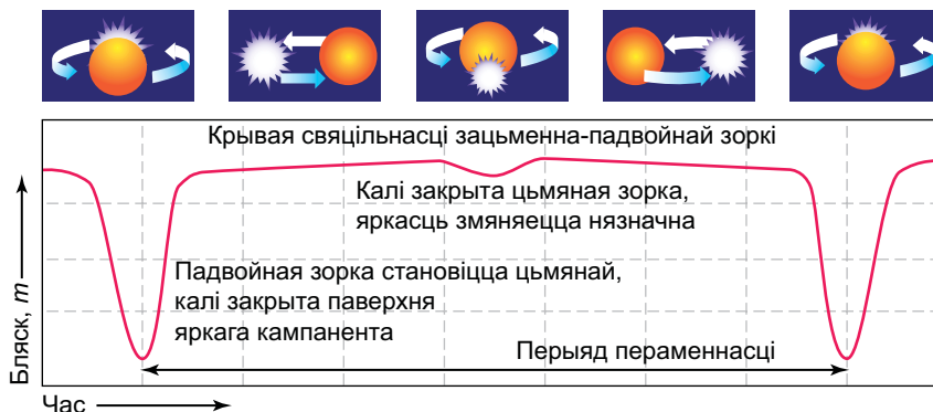
Рыс. 125. Змяненне бляску зацьменна-падвойнай зоркі
