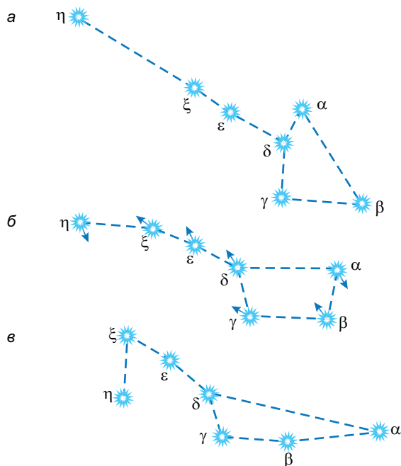
Рис. 146. Змяненне адноснага размяшчэння зорак у «каўшы» Вялікай Мядзведзіцы за 100 тыс. гадоў: а — 50 тыс. гадоў назад; б — наш час (стрэлкамі паказаны напрамкі тангенцыяльных скарасцей зорак); в — праз 50 тыс. гадоў
