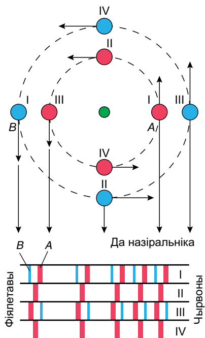
Рыс. 126. Зрушэнне ліній у спектры падвойнай зоркі
