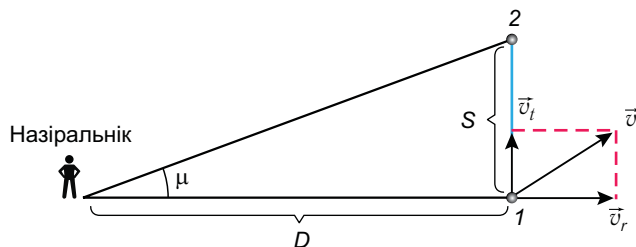
Рис. 145. Вызначэнне тангенцыяльнай скорасці зоркі
