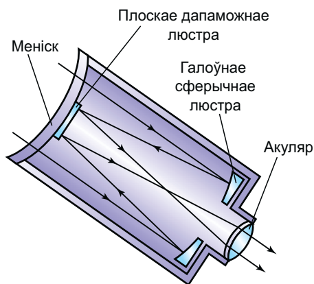
Рыс. 99. Ход праменяў у люстрана-лінзавым меніскавым тэлескопе
