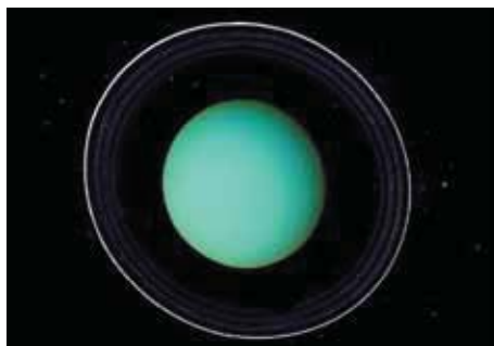
Рис. 69. Уран. Фатаграфія атрымана касмічным тэлескопам Хабла
