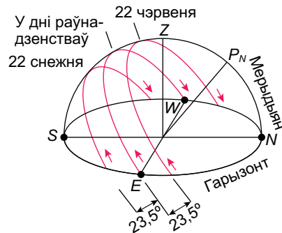
Рыс. 29. Сутачныя шляхі Сонца над гарызонтам у розныя поры года пры назіраннях у сярэдніх геаграфічных шыратах
