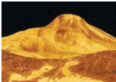
Рис. 55. Гора Маат — патухлы вулкан на Венеры
