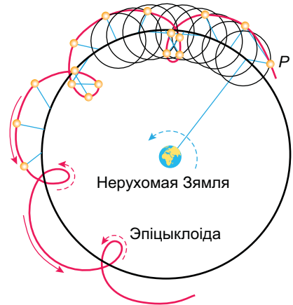
Рис. 24. Траектория планеты по вавле тэорыі Пталемея
