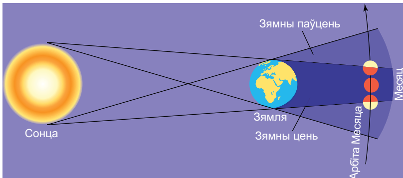
Рыс. 34. Схема месяцовага зацьмення
