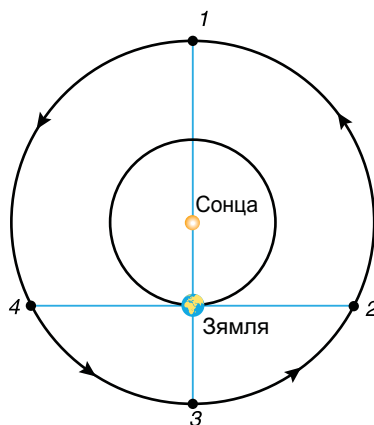
Рыс. 27. Схема канфігурацый верхніх планет: 1 — злучэнне; 2 — заходняя квадратура; 3 — процістаянне; 4 — усходняя квадратура
