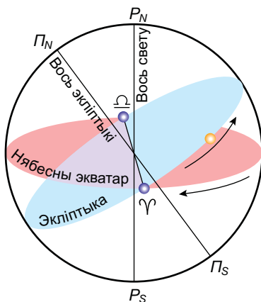
Рыс. 13. Экліптыка
