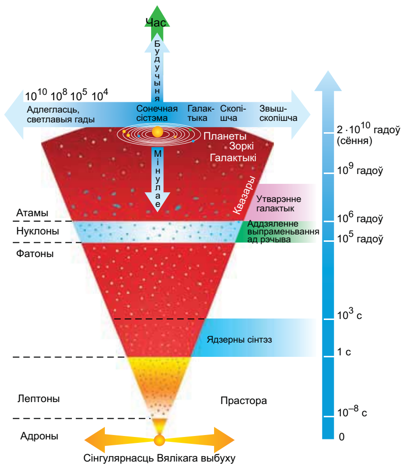
Рис. 169. Схема развіцця Сусвету ад Вялікага выбуху да нашага часу
