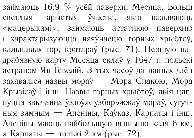
Рис. 71. Выгляд месяца ў тэлескоп
