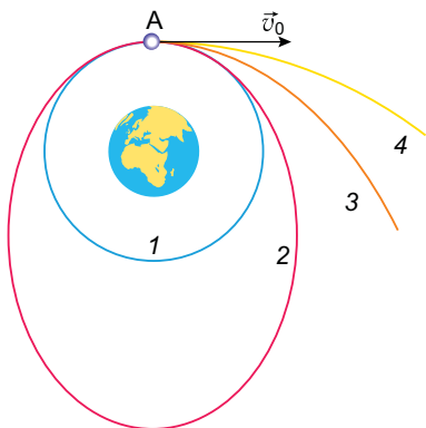
Рис. 47. Формы арбіт касмічных апаратаў: 1 — кругавая; 2 — эліптычная; 3 — парабалічная; 4 — гіпербалічная
