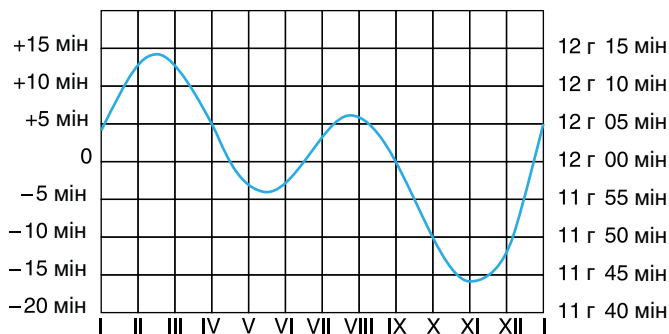
Рыс. 19. Графік ураўнення часу
