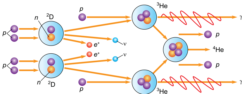
Рис. 111. Схема пратон-протоннай рэакцыі: p — пратон; n — нейтрон; ^2\text{D} — ядро дэйтэрыю; ^3\text{He} , ^4\text{He} — ядры ізатопаў гелію; e^+ — позитрон; \nu — нейтрына; \gamma — гама-квант
