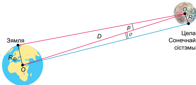
Рис. 44. Вызначэнне лінейных памераў цел Сонечнай сістэмы
