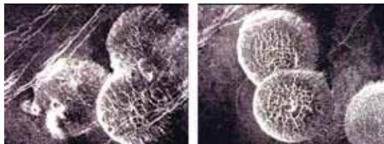
Рис. 56. Застылыя пузыры вулканічнай лавы на Венеры. Радыёлакацыйны відарыс, перададзены касмічным караблём «Магелан» у 1991 г.
