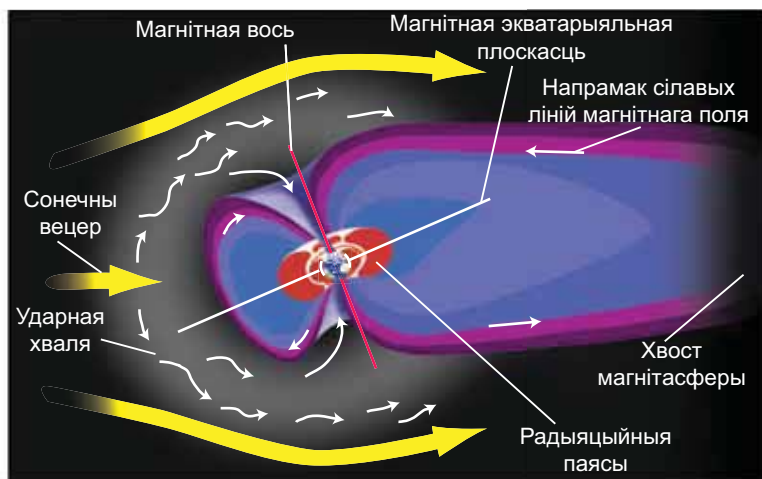
Рис. 120. Схема ўтварэння магнітасферы Зямлі
