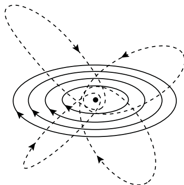
Рыс. 147. Траекторыі зорак у Галактыцы (дыск Галактыкі — сцэльныя лініі, сфэрычная складальная — пункцірныя лініі)
