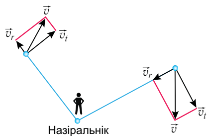
Рыс. 144. Прастарава ( v ), прамянёвая ( v_r ) і тангенцыйная ( v_t ) скорасці
