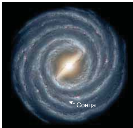
Рыс. 141. Будова нашай Галактыкі. Стрэлка паказвае месцазнаходжанне Сонечнай сістэмы
