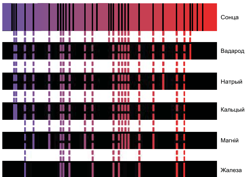
Рыс. 109. Адпаведнасць паміж месцазнаходжаннем фраўнгоферавых ліній сонечнага спектра і ліній хімічных элементаў
