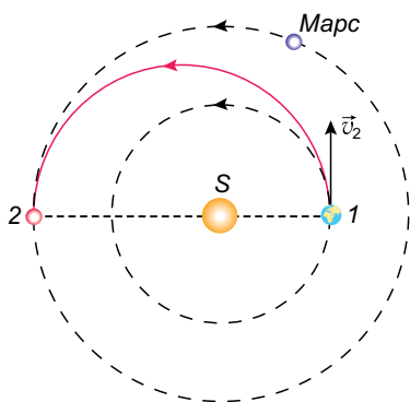
Рис. 48. Гоманайская траекторыя пералёту з Зямлі на Марс
