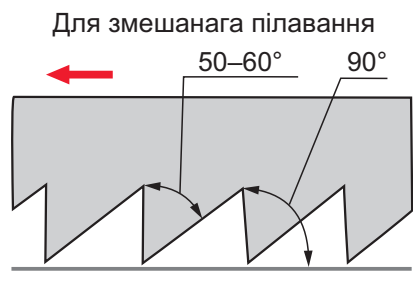
Мал. 20. Зубы піл
