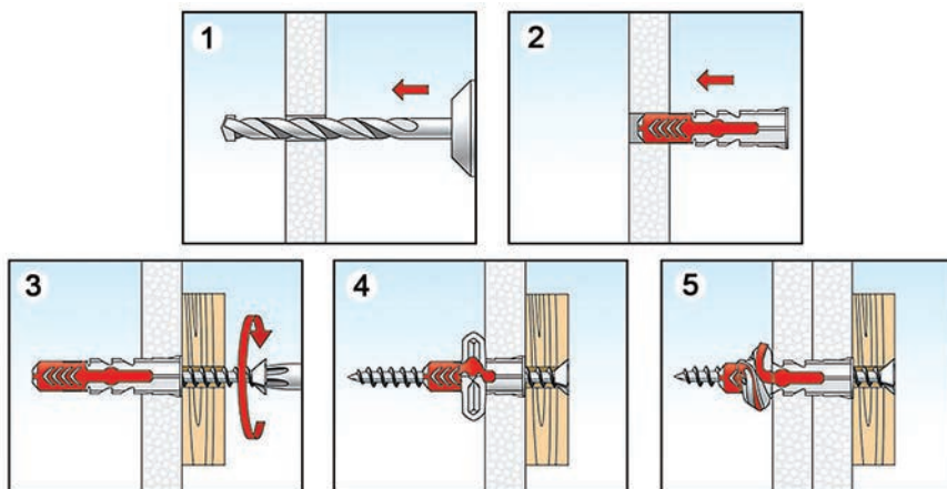
Мал. 139. Мацаванне прадмета з дапамогай універсальнага дзюбеля
