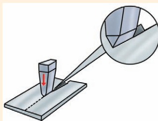
Мал. 101. Становішча рэжучай часткі зубіла пры рубцы
