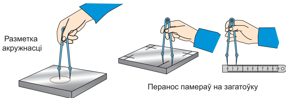
Мал. 93. Разметка цыркульем
